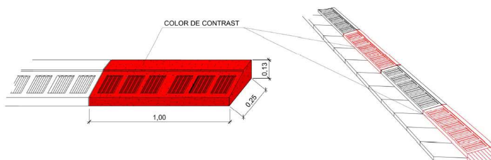
Imatge 1. Vorada remuntable amb franges blanques i de color vermell (cotes en m).
