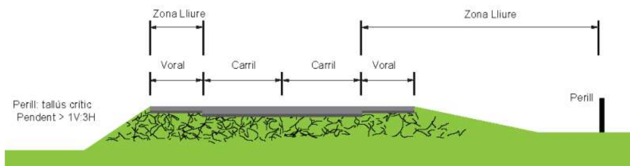
Imatge 1. Zona Lliure d'una carretera.
