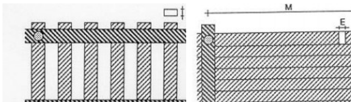
Exemple d'estrebat vertical semi-quallat (esquerra) i quallat (dreta)
