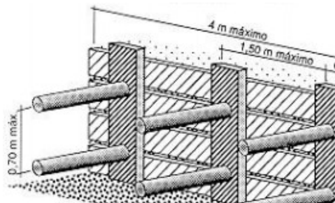
Exemple d'estrebat horitzontal
