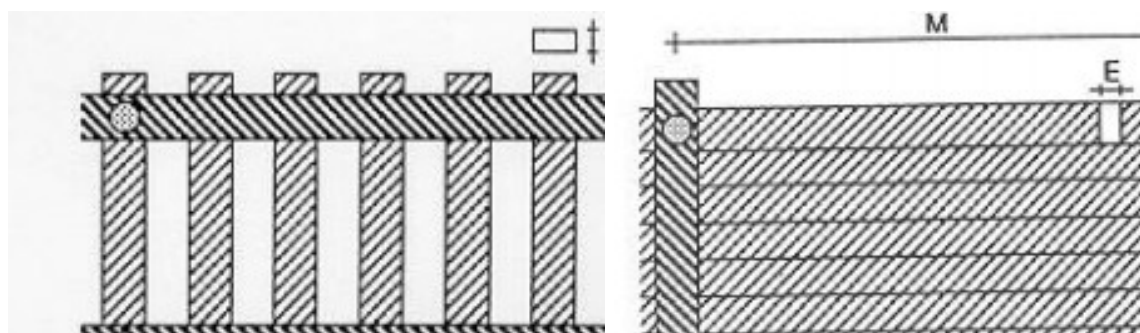
Exemple d'estreat vertical semi-quallat (esquerra) i quallada (dreta)
